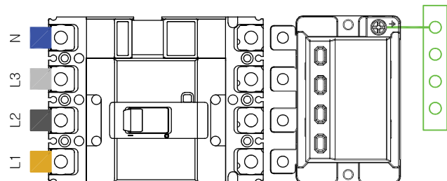
3 Phase 4 Wire 3상 4선
